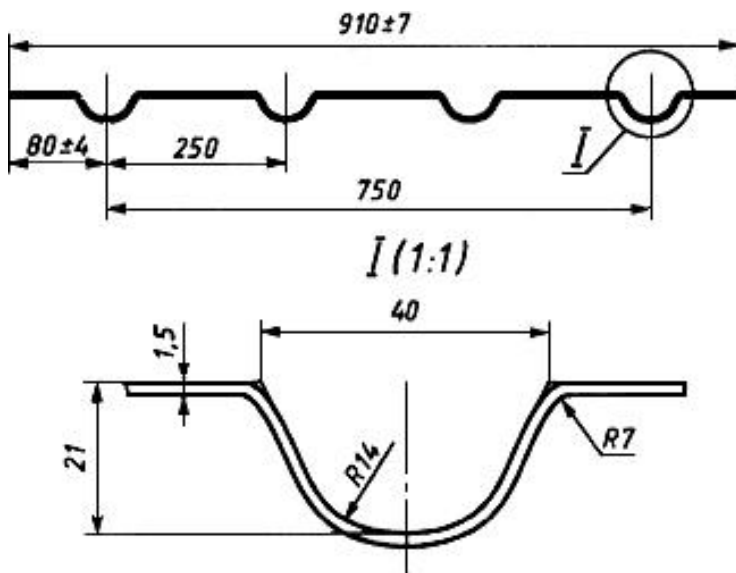
Рисунок 5 - Профиль 940x22,5x1,5, ГЛ4-216
