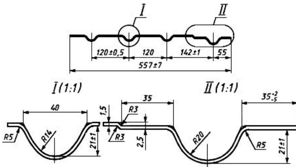
Рисунок 4 - Профиль 557x21x1,5, ГЛ4-238
