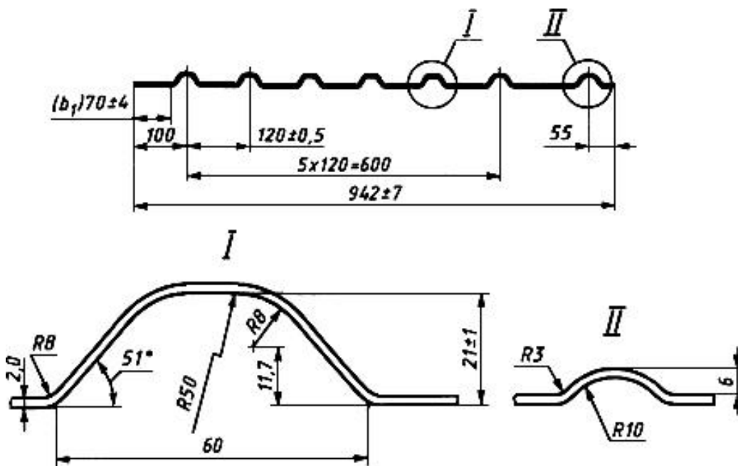
Рисунок 3 - Профиль 942x21x2,0, ГЛ4-221; профиль 940x21x2,0 ГЛ4-231
