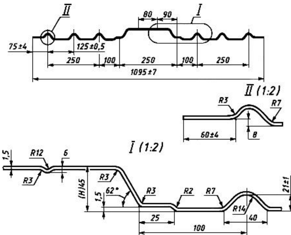
Рисунок 2 - Профиль 1095x45x21x1,5, ГЛ4-220А
