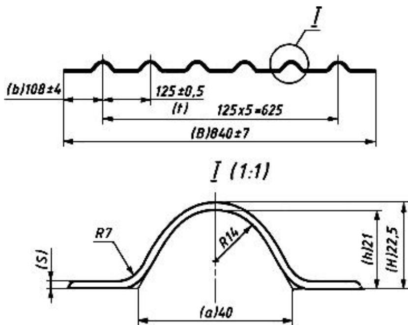
Рисунок 1 - Профиль 840x21x1,5, ГЛ4-218; профиль 840x21x2,0, ГЛ4-219
